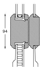
VANDRET
