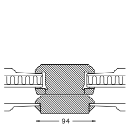
LODRET
